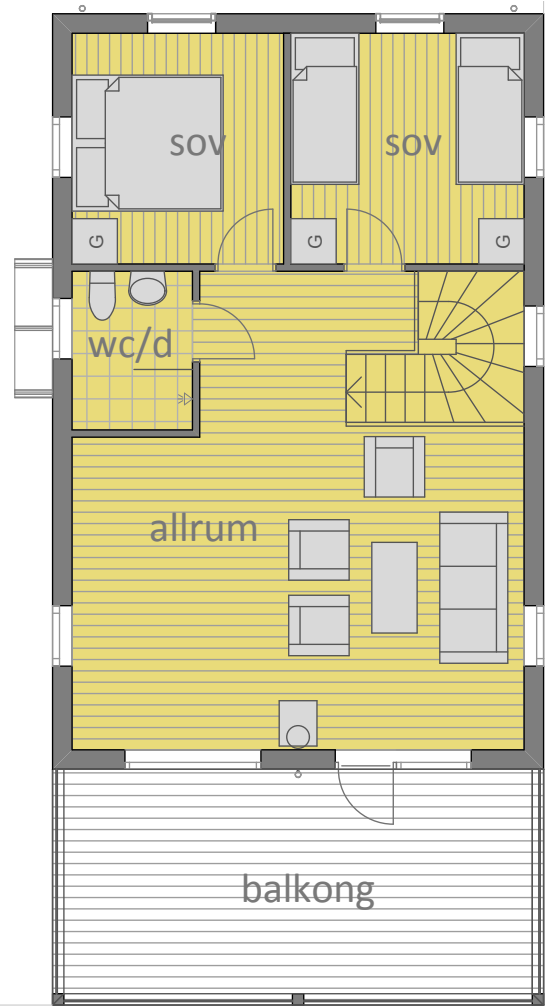
Övervåning
