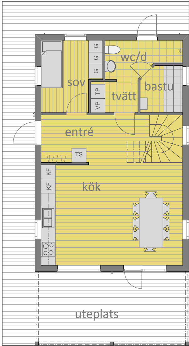
Entréplan
